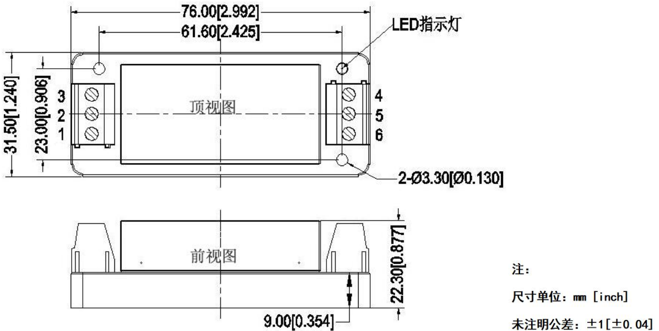
引脚定义
