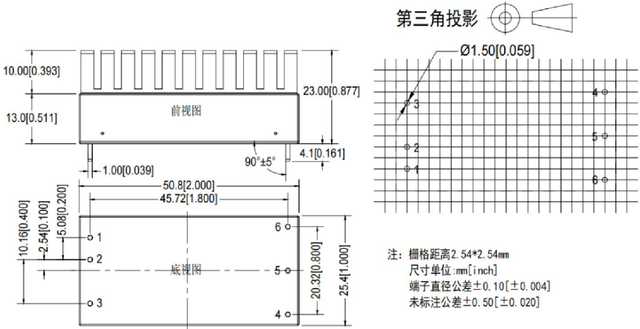
引脚定义
